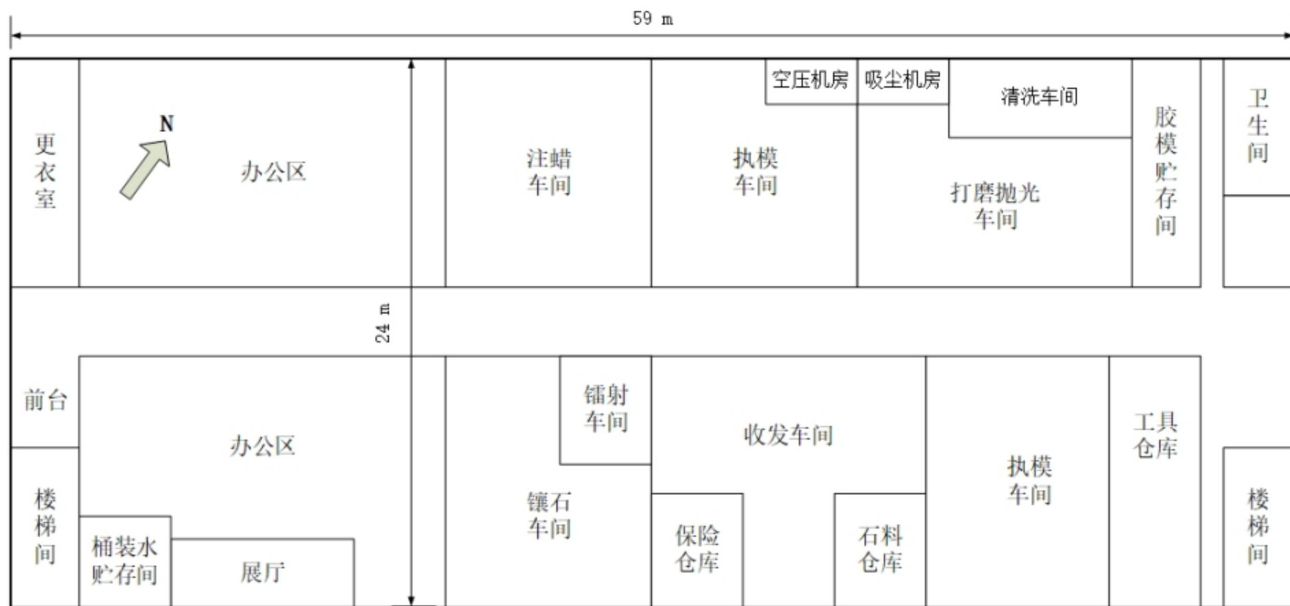
图 3-3 项目平面布置图
